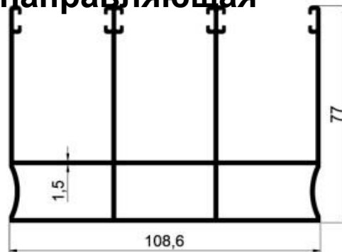
Боковая направляющая
