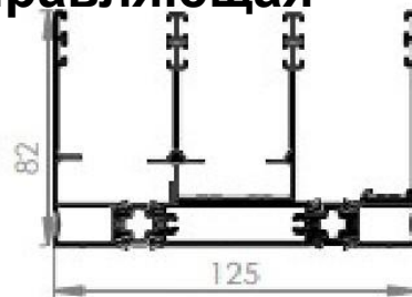
Боковая направляющая
