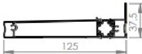
Нижняя направляющая
