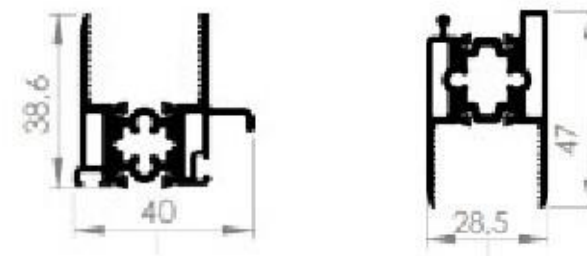
Створочный профиль
